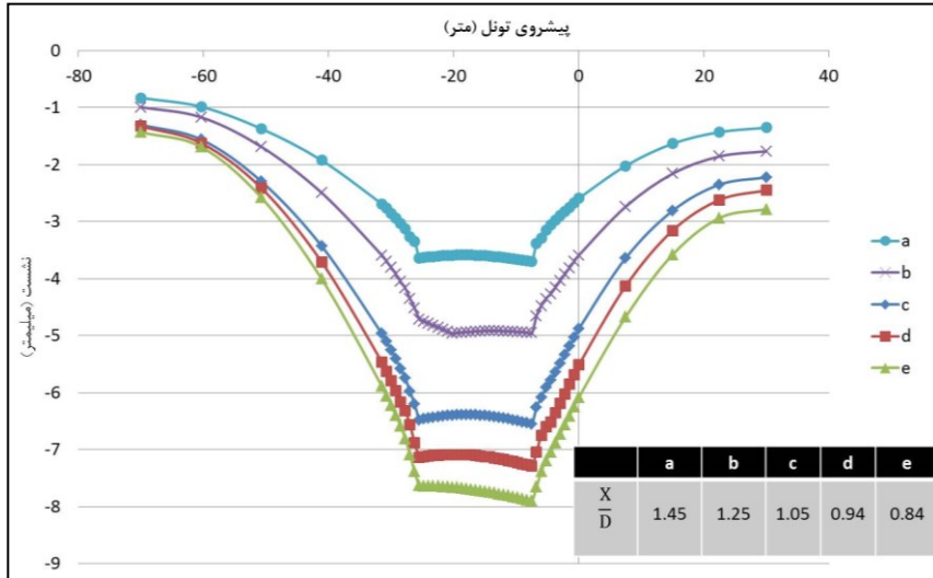
شکل ۵: تغییرات منحنی نشست طولی به ازای تغییر نسبت \frac{X}{D} و در زیر مرکز ثقل سازه.
