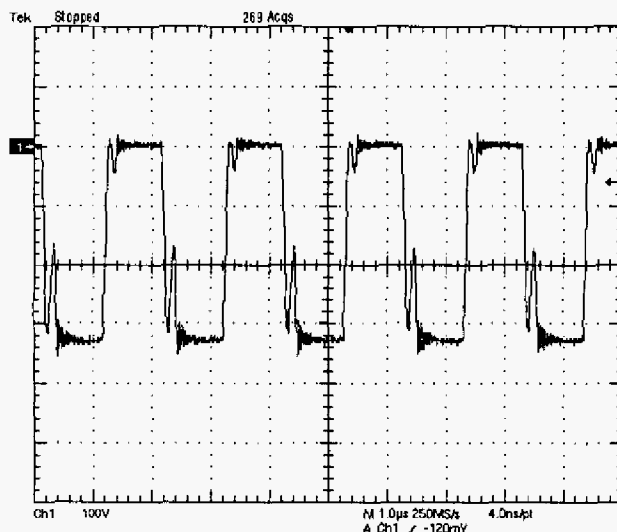
Fig. 12. Diode voltage
