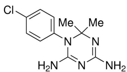
Cycloguanil
